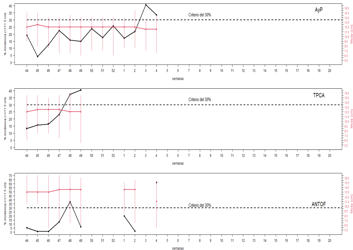
Figura 3. Variabilidad semanal de la incidencia de ejemplares juveniles (línea negra) y de la moda (con amplitud de tallas (cm) en línea vertical roja), por región. La línea horizontal punteada: criterio 30% de activación de veda.
